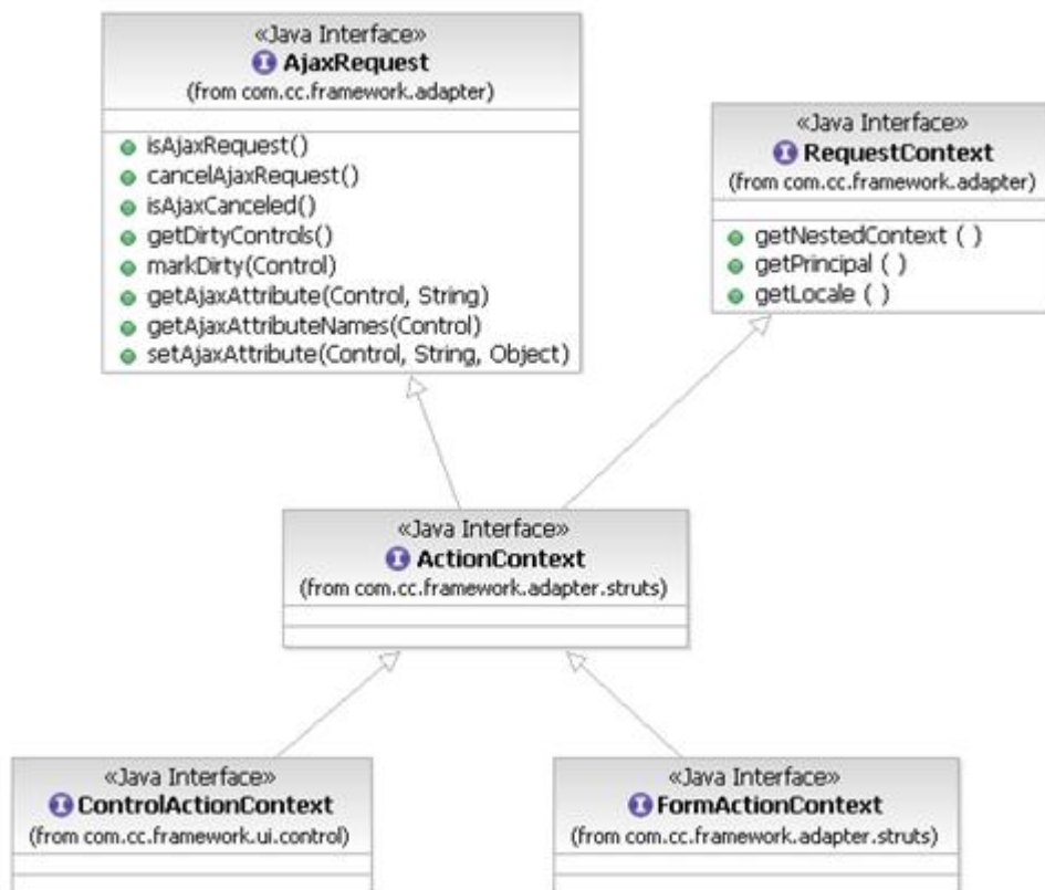
Abbildung 2: Vererbungshierarchie ActionContext
